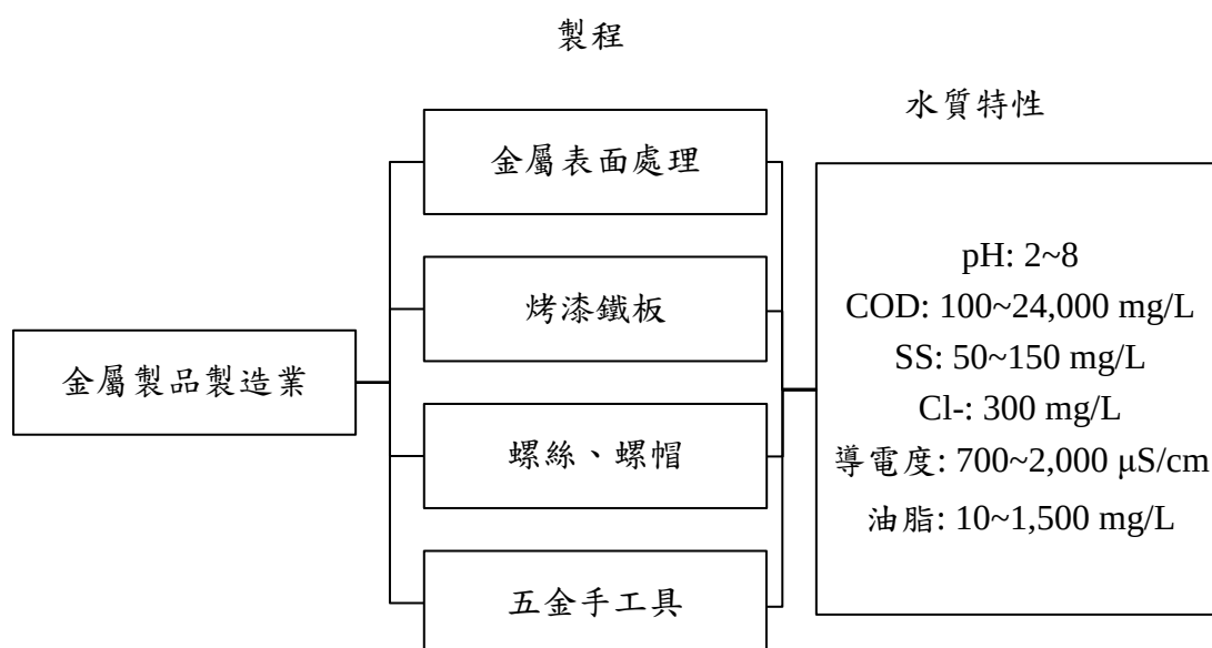
圖 6 金屬製品製造過程所產生廢水水質特性
