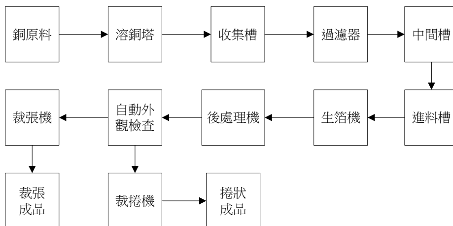
圖 36 案例 A 廠生產製造流程圖
