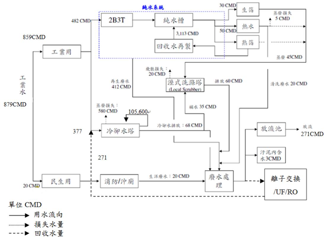
圖 38 案例 A 廠用水平衡圖（方案實施後）
