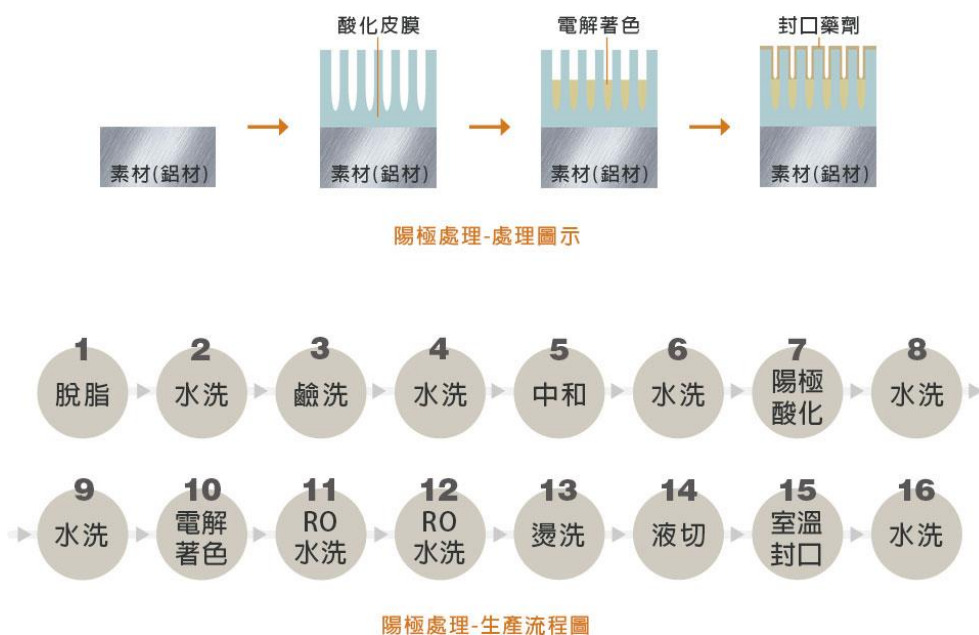
圖 4 金屬加工處理業作業流程（以金屬表面處理為例）
