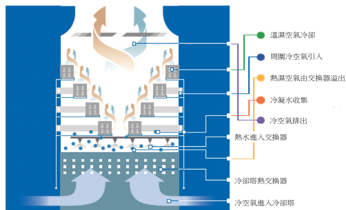
圖 21 冷卻水塔蒸發回收系統圖
