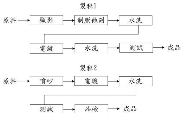
圖 39 案例 B 廠製造流程圖
