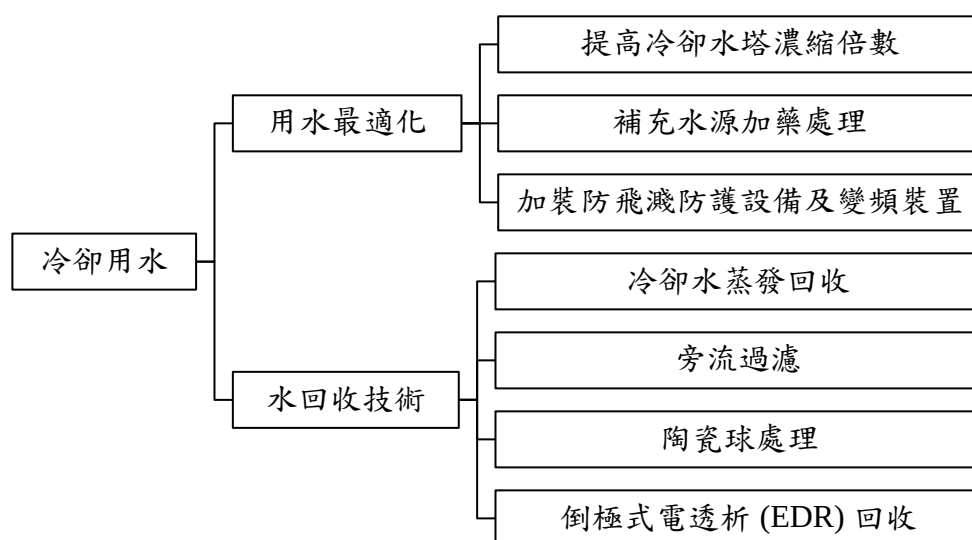
圖 17 冷卻用水最適化以及水回收技術
