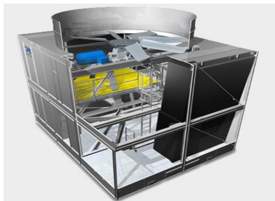
圖 21 冷卻水塔蒸發回收系統圖
