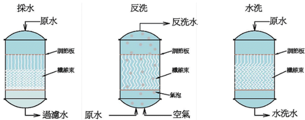
圖 9 纖維過濾設備原理
