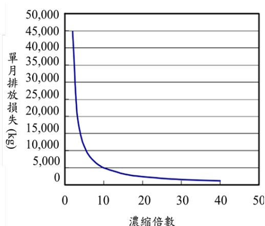
圖 10 濃縮倍數與排放損失關係圖
