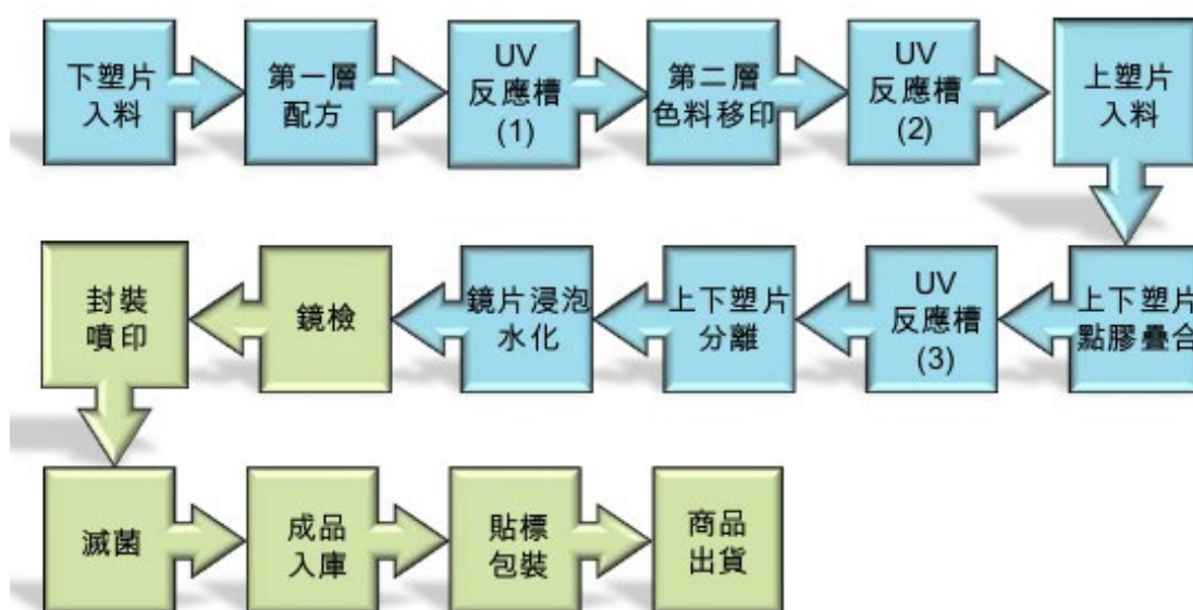
圖 4 隱形眼鏡製造流程圖
