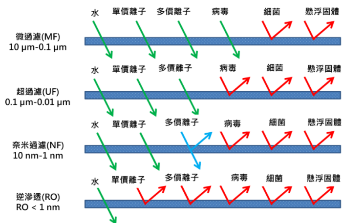
圖 24 各種濾膜去除物質比較
