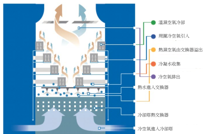
圖 13 冷卻塔蒸發回收系統圖
