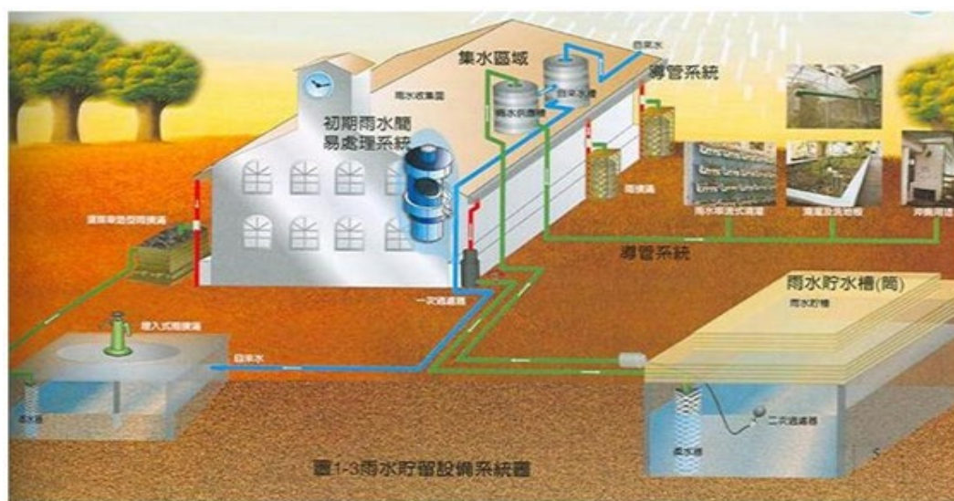
圖 38 雨水載流設備系統圖
