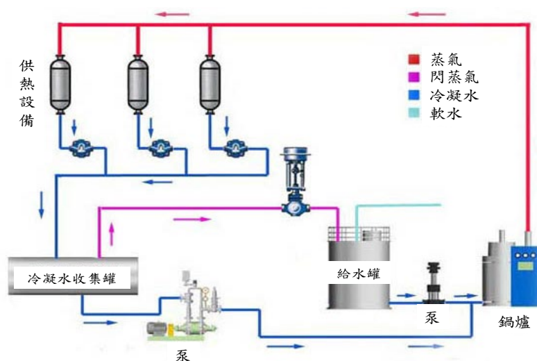
圖 22 密閉式冷凝水回收系統示意圖
