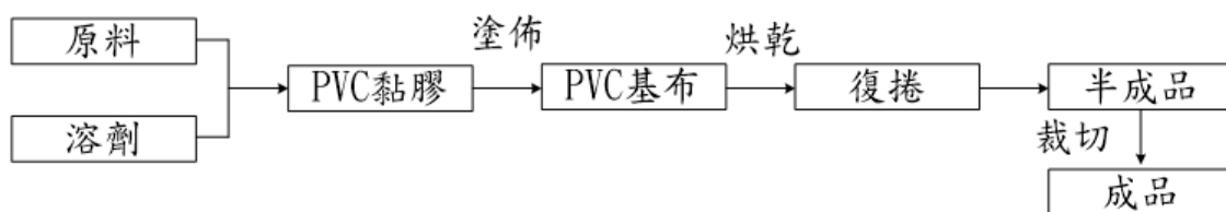
圖 35 案例 A 廠製程流程圖
