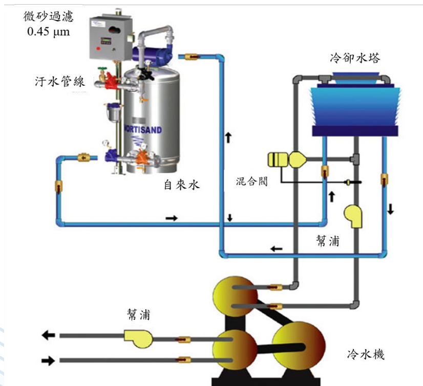
圖 15 旁流過濾處理系統原理示意圖
