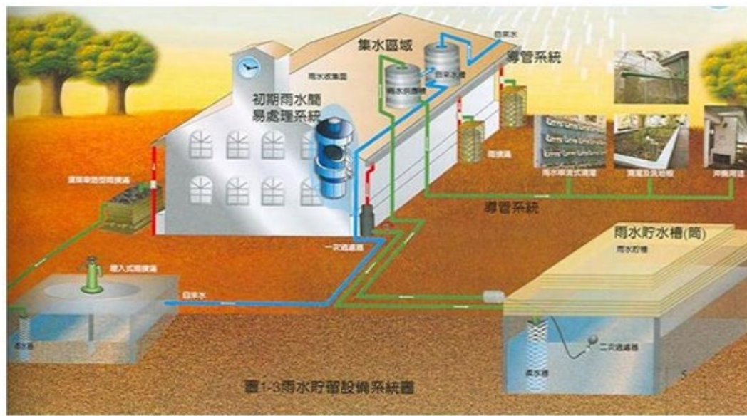
圖 42 雨水載流設備系統圖
