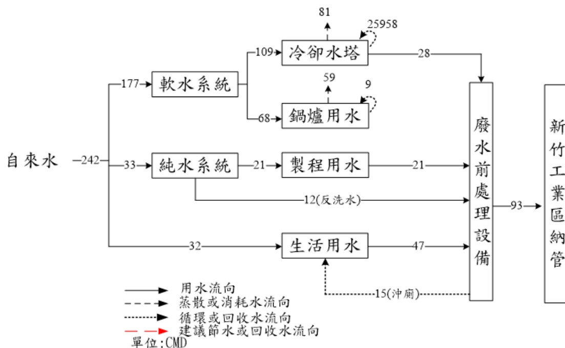
圖 36 案例 A 廠用水平衡圖（方案實施前）
