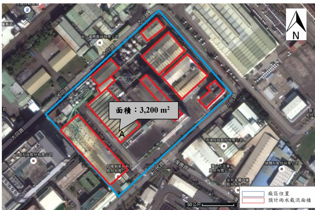
圖 37 雨水收集區示意圖
