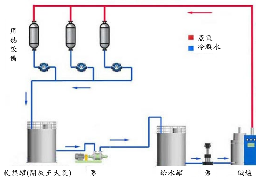
圖 21 開放式冷凝水回收系統示意圖
