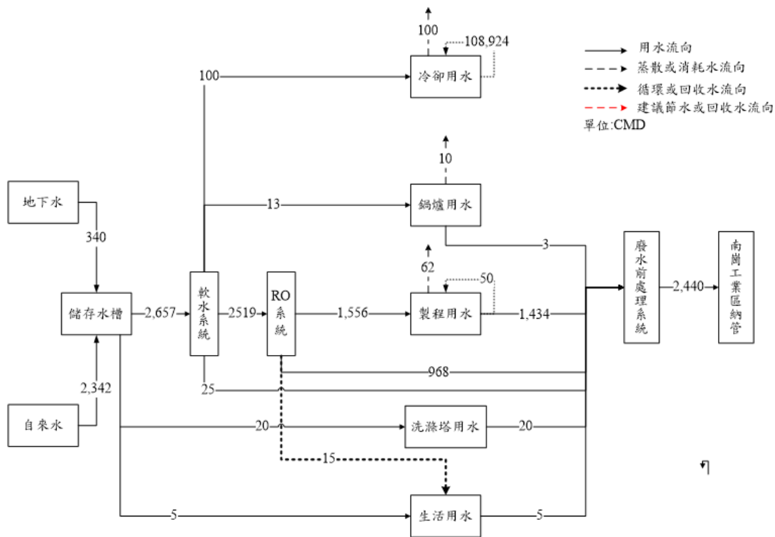
圖 41 案例 B 廠用水平衡圖（方案實施前）
