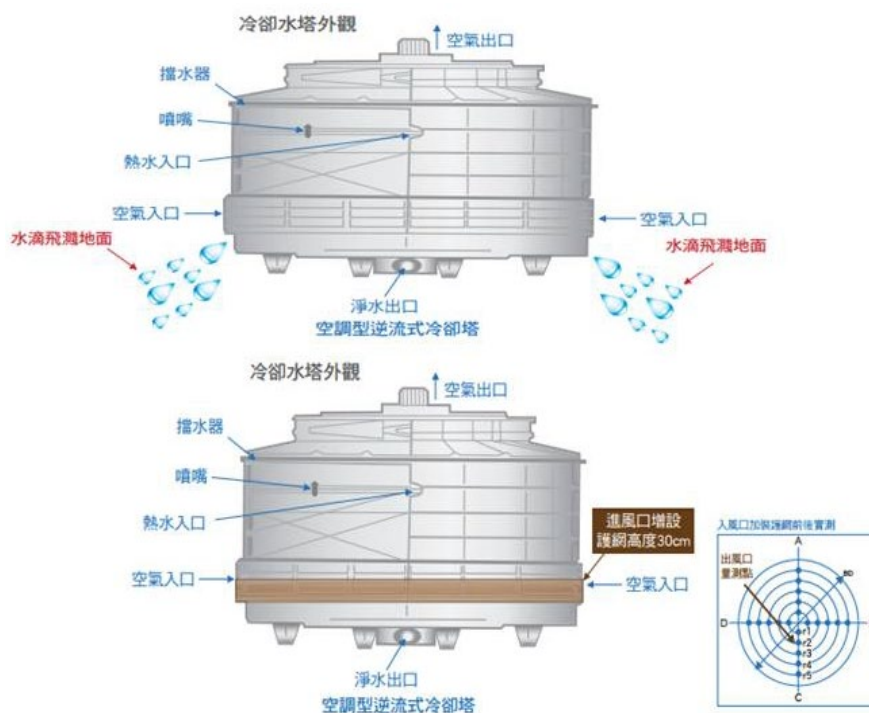
圖 12 冷卻水塔防飛濺防護設備圖
