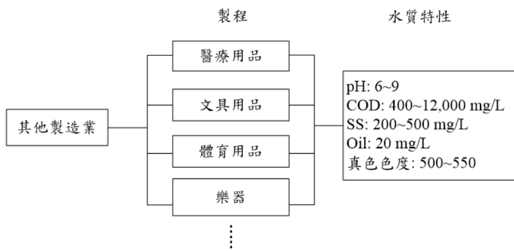
圖 6 其他製造業製程廢水特性
