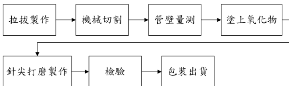
圖 3 針頭製造流程圖
