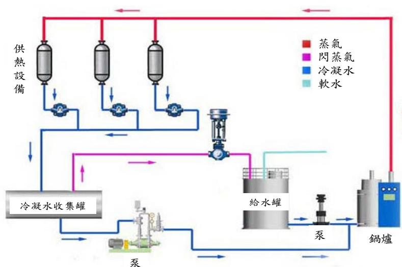
圖 20 密閉式冷凝水回收系統示意圖
