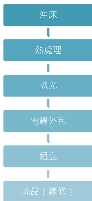
圖 2 自行車鍊條製造流程圖
