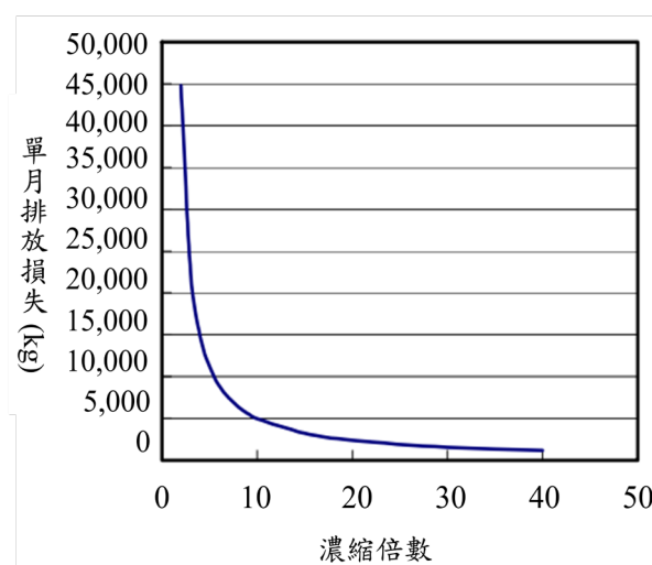
圖 8 濃縮倍數與排放損失關係圖
